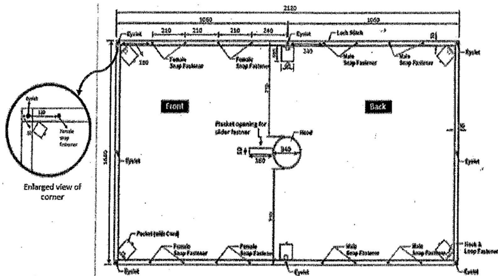
Fig: 3A Poncho (Outerview)
