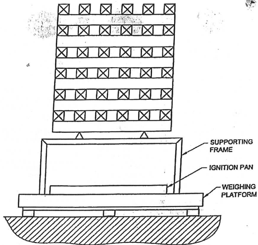
FIG. 2 CRIB FIRE
